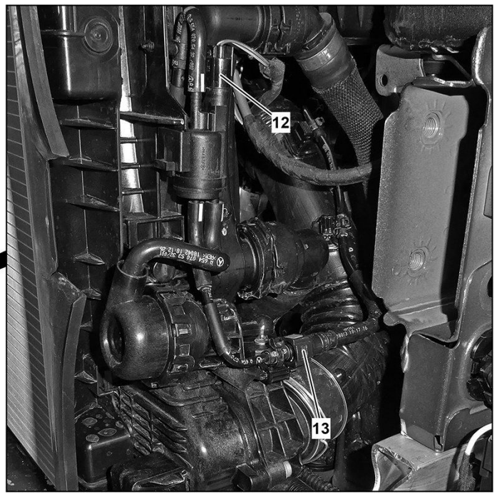
13 Unterdruckleitung
